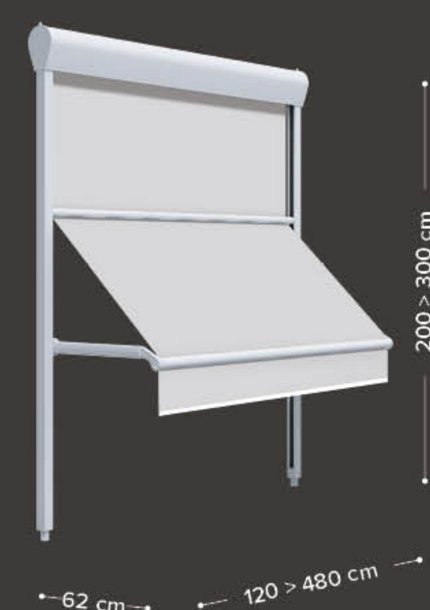
DIM 6 senza cassonetto / without cassette
